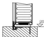
Anschlag mit Dichtung
