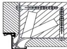
Einbau mit Mauer-Dübelanker
